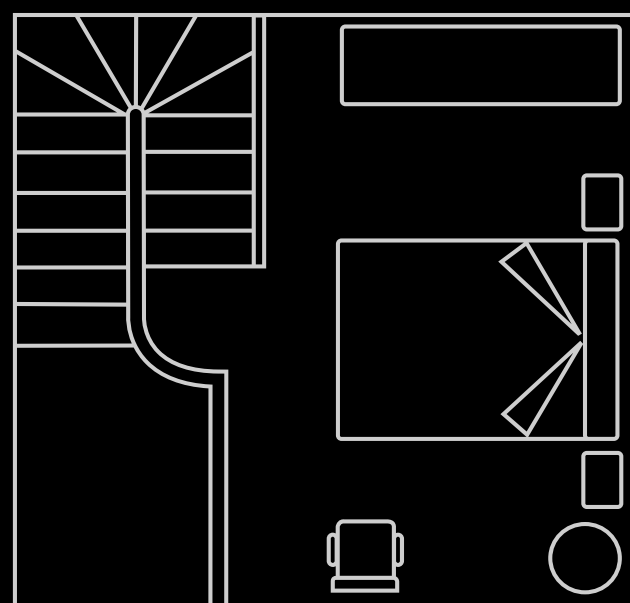
Planta 2 Dormitorio: 15 m²
